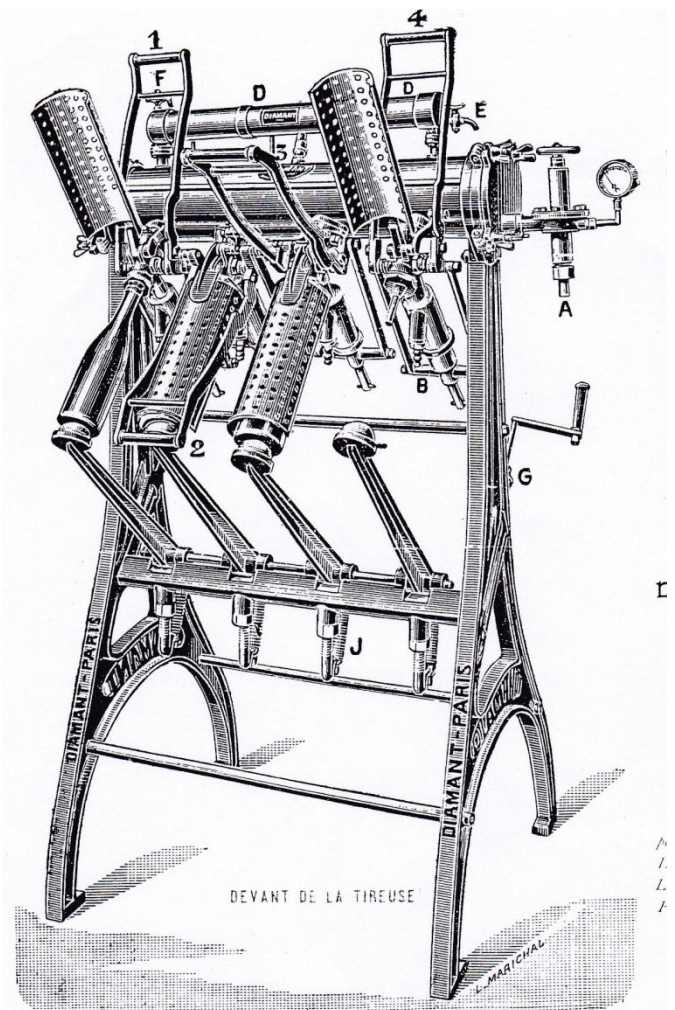
Tireuse doseuse Diamant
